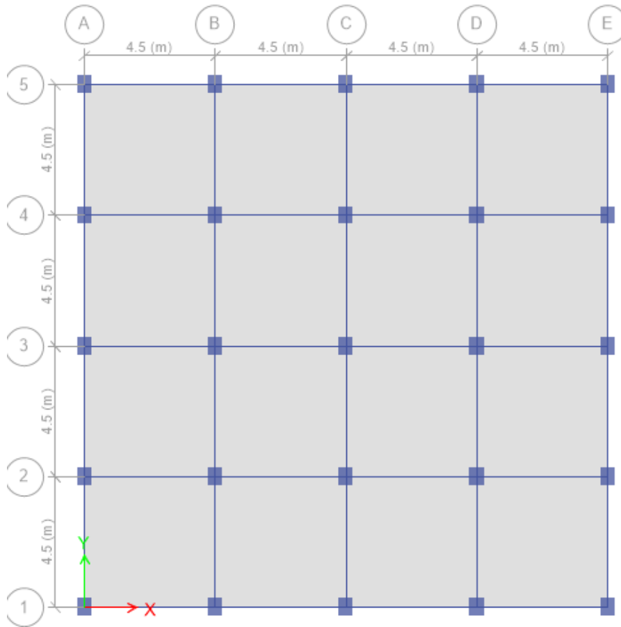
Fig. 1 Plan
