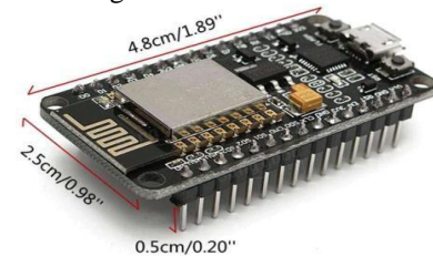
Fig. 6: Node MCU
