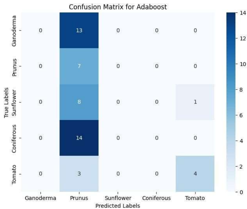
Fig 10. Adaboost Output
