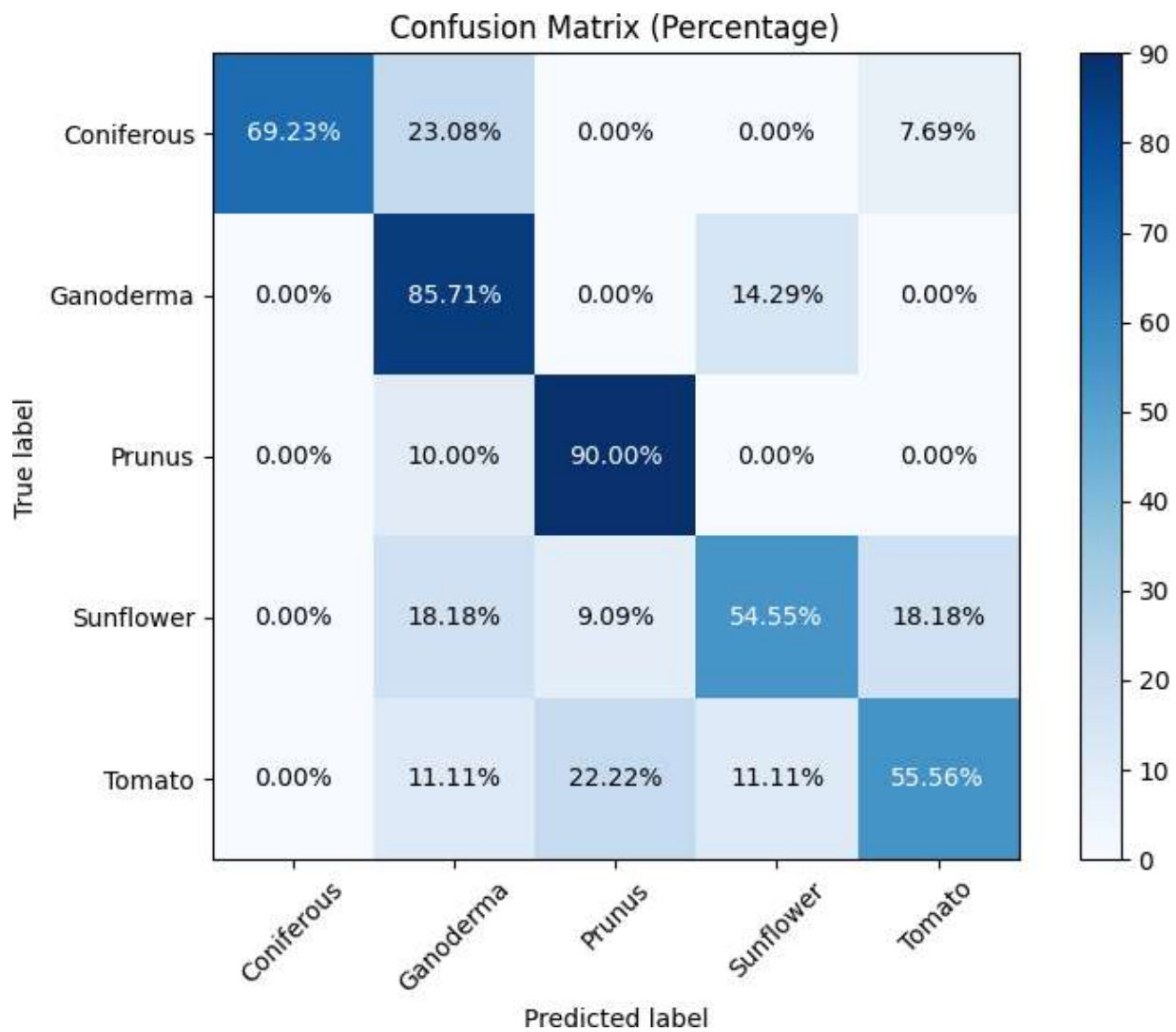
Fig 8. SVM Output
