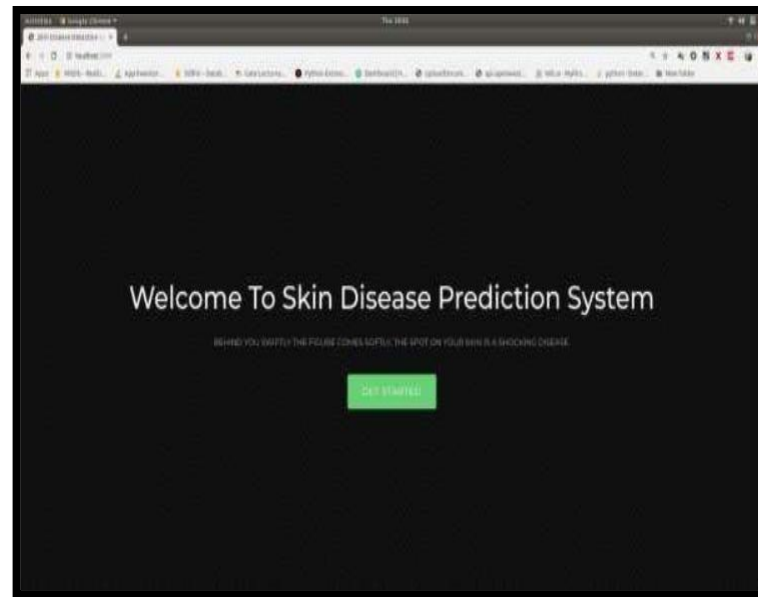
fig-4:welcome page.
