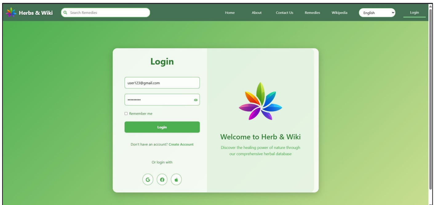
Figure4: Login Page
